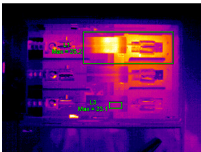
3-fázisú biztosíték túlmelegedése
