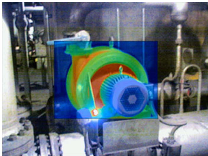
Kép a képben IR-Fusion csökkentett infra telítettséggel
