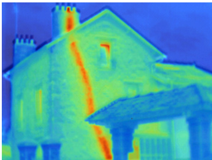
Hővesztés a kéményen keresztül
