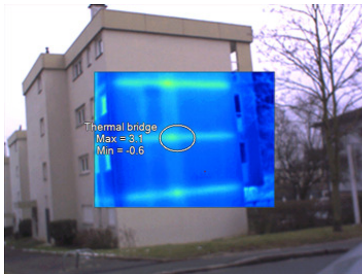
Épület hőhidak
