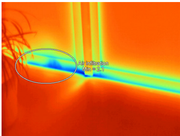
Levegő beszivárgás üvegajtónál
