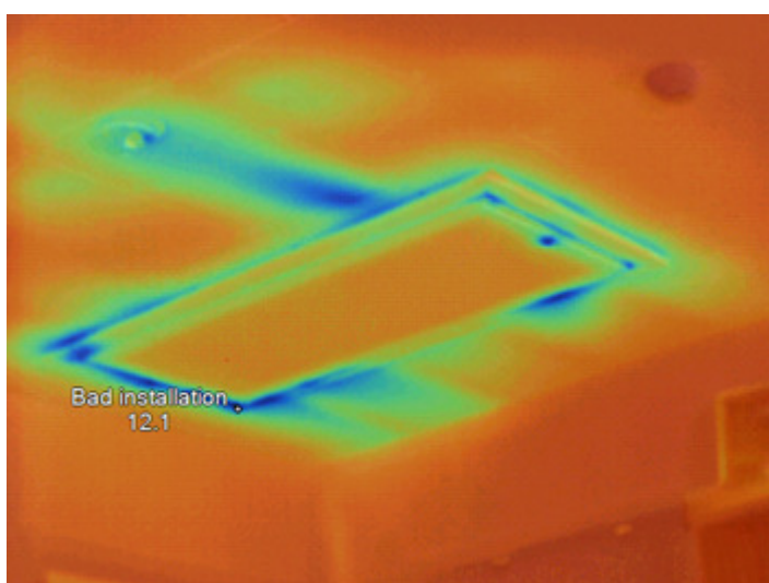
Padlásszoba feljáró, hideg levegő beszivárgás
