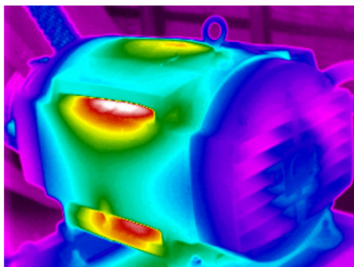
Abnormális, egyenetlen melegedés motornál
