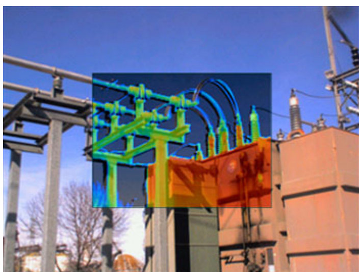
IR-Fusion kép csökkentett infra telítettséggel
