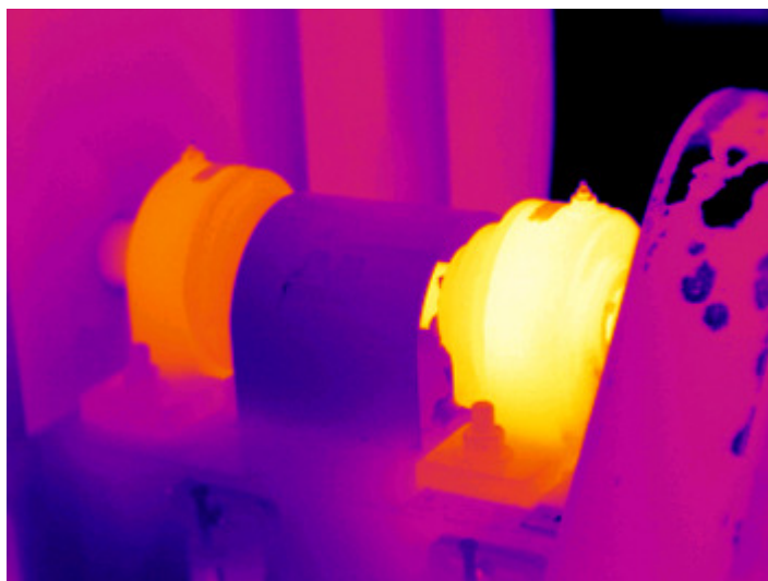
Túlmelegedett csapágyház
