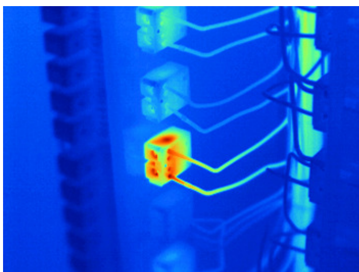
Túlterhelt világításvezérlő áramkör
