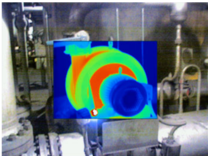
Kép a képben IR-Fusion
