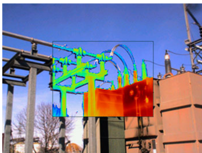
IR-Fusion kép látható riasztással
